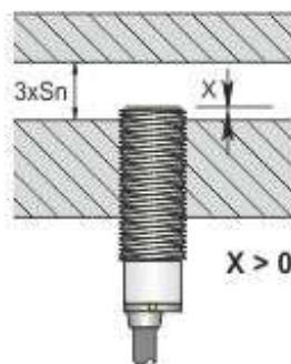
Montaje enrasado
